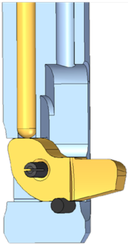
BSF-P: Il bullone di bloccaggio aggiuntivo nell'alloggiamento lama consente di posizionare la lama con maggiore precisione.
