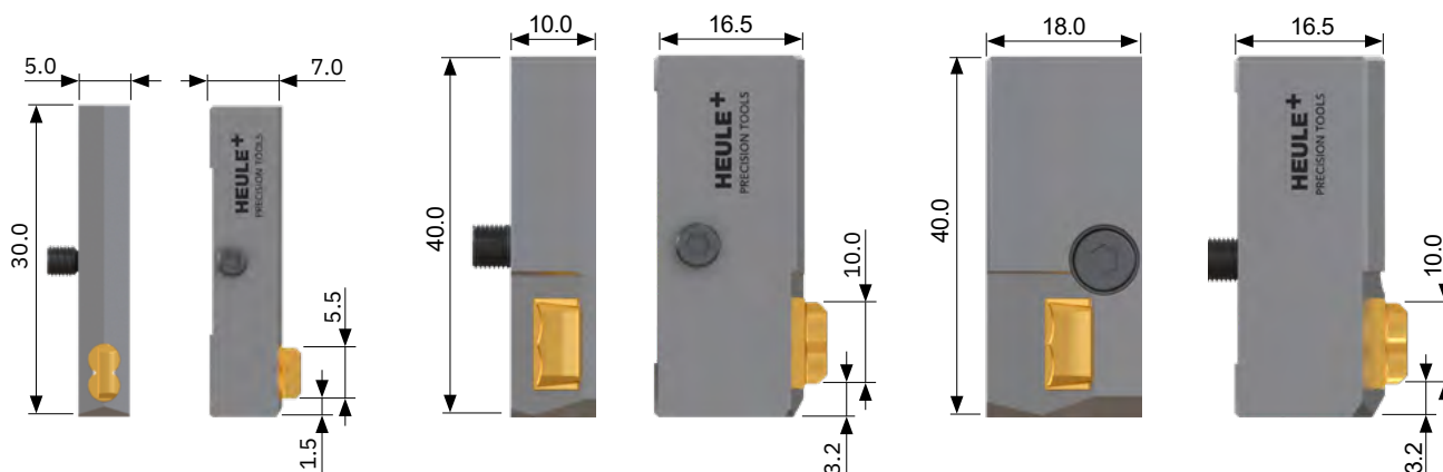
SNAP5 >Ø12.6
