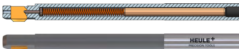
Sistema de cartuchos
