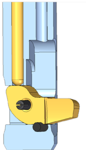
BSF-P: Il bullone di bloccaggio aggiuntivo nell'alloggiamento lama consente di posizionare la lama con maggiore precisione.
