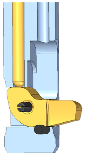
BSF-P : Le piolet de blocage supplémentaire dans le porte-couteau permet un positionnement plus précis du couteau.
