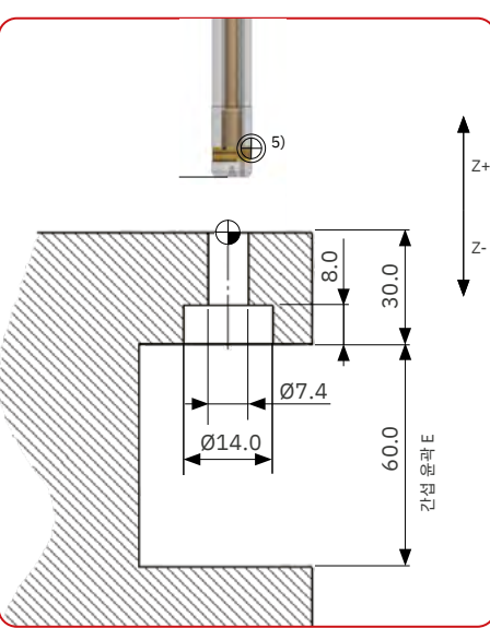
보어 뒷면의 실린더 카운터 싱크
